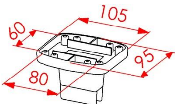
Befestigungsplatte MOVE mounting plate MOVE
